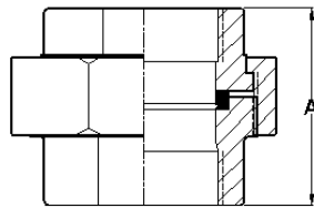
Fig. 830 B
